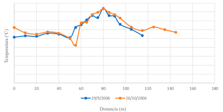
Figura 2. Periodo de mediciones de temperatura en el perfil sur-este del cráter del VSA, entre los meses de septiembre y octubre de 2006.
