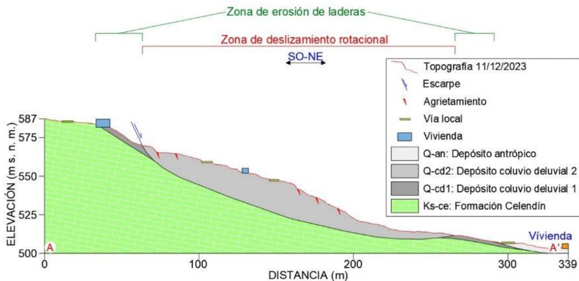
Figura 11. Perfil longitudinal A-A' donde se aprecia la distribución de los materiales geológicos del deslizamiento de San Luis Alto.
