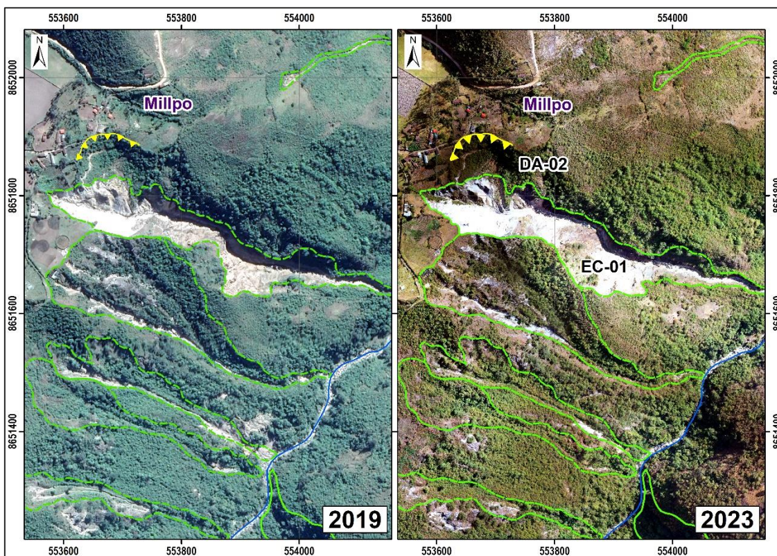
Figura 16. Comparación multitemporal de una imagen satelital (2019) y el ortomosaico actual, obtenido mediante sobrevuelos de dron (2023), donde se puede visualizar el avance de la erosión en cárcava.
