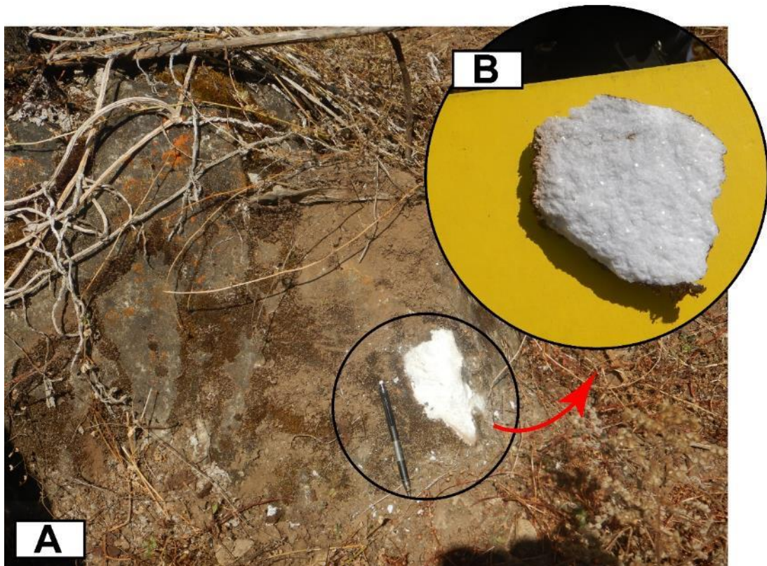
Figura 6. A. Vista de una roca intrusivas de naturaleza monzogranítico, observado en los alrededores de la zona evaluada. B. Muestra de mano, donde se evidencia la textura gruesa y los cristales bien desarrollados de color blanco lechoso, producto de la gran cantidad de cuarzo que presenta la roca.
