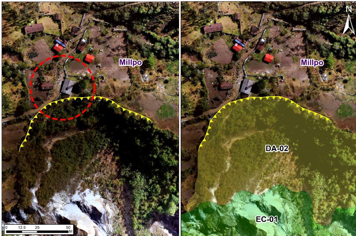
Figura 13. Deslizamiento activo DA-02 , ubicado en el sector Millpo, condicionado principalmente por el avance progresivo de la erosión en cárcava ( EC-01 ) ubicado al pie deslizamiento y que pone en riesgo a viviendas ubicadas cerca del escarpe principal.
