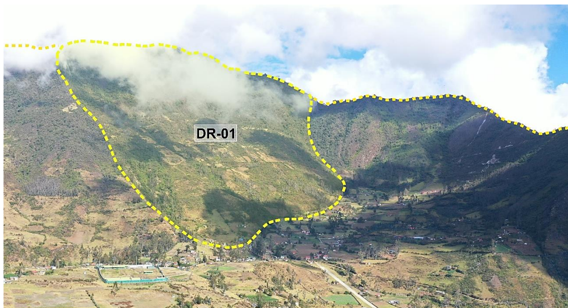
Figura 10. Vista del deslizamiento reactivado DR-01 , con un área aproximada de 99 ha y caracterizado por un escarpe principal de forma irregular y continua de 1300 m de longitud. Actualmente se desarrolla actividades de cultivos sobre el cuerpo deslizado.
