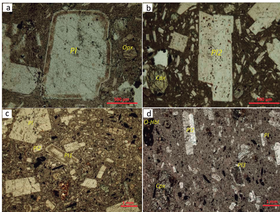
FIGURA 2. Microfografías texturas celulares en plagioclasas del Volcán Nevado del Ruiz. a) muestra una población de plagioclasas (P11) con núcleos y bordes limpios y una franja concéntrica con textura celular fina; b) se indica una población de cristales de plagioclase (P12) con textura celular gruesa en el núcleo con un borde extremo limpio; c) poblaciones de plagioclasas con diferentes texturas de corrosión (P11 y P12), y cristales limpios (P1); d) muestra un tercer tipo de textura en donde el núcleo se encuentra totalmente corroído con textura celular fina (P13).
