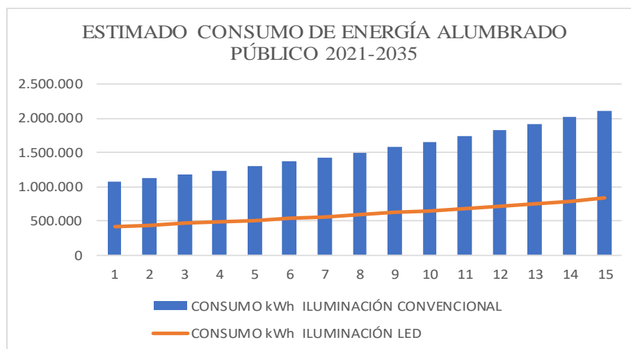
Figura 1. Comparativo alumbrado público tecnologías convencionales y LED.
