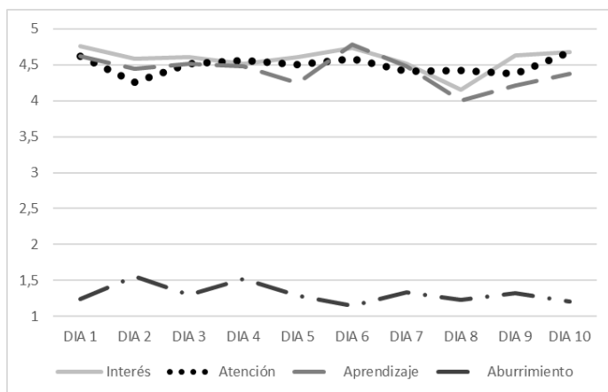
Figura 1. Seguimiento de la valoración de la asignatura diana en cuanto al interés, atención, aprendizaje y aburrimiento percibido por los estudiantes
