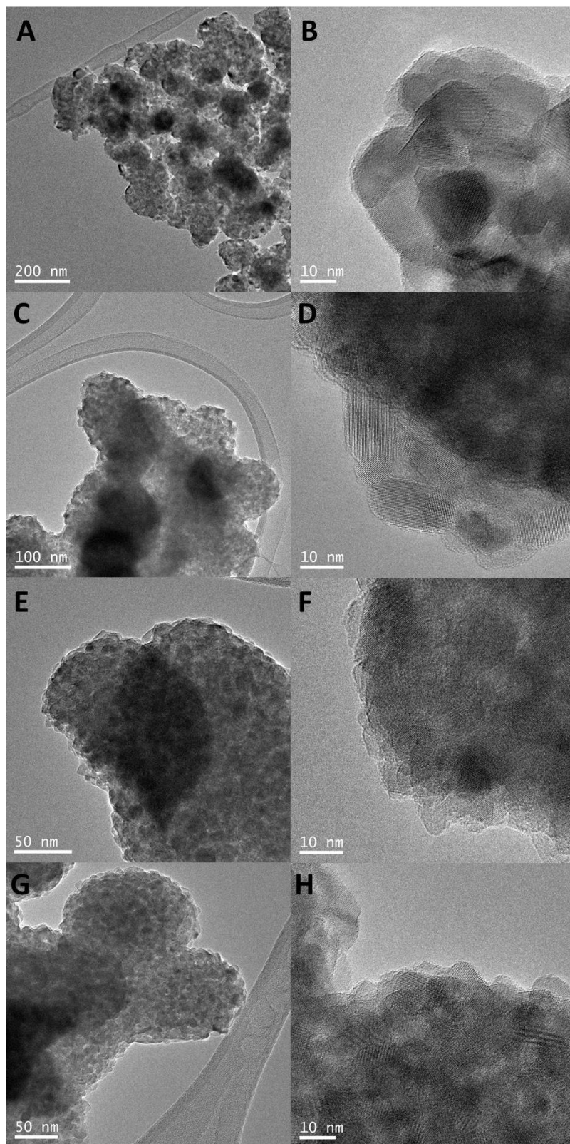
Figure 3. TEM images of the TiO 2 reference (A-B), TiO 2 -TPA10 (C-D), TiO 2 -TPA20 (E-F) and TiO 2 -TPA30 (G-H) samples.
