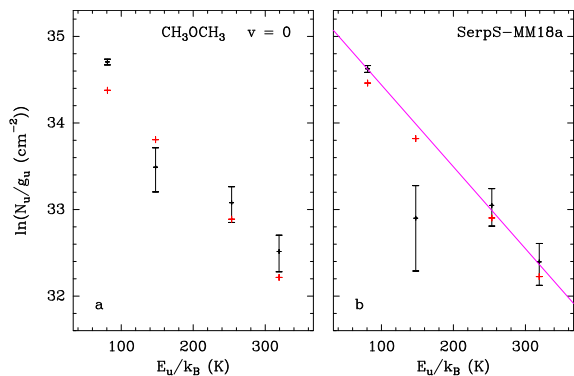
Fig. E.62. Same as Fig. E.1 but for CH 3 OCH 3 in SerpS-MM18a.
