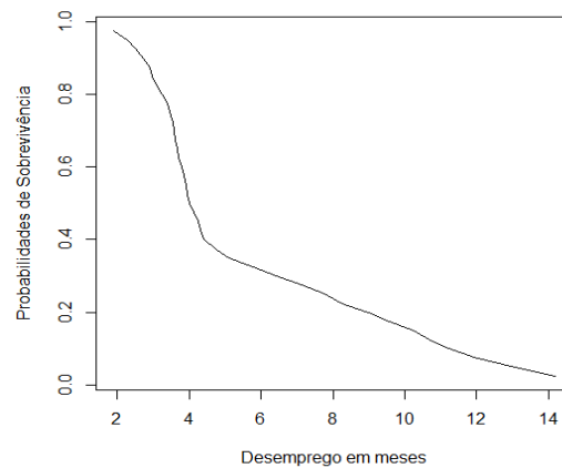
Gráfico 3: Função de Sobrevivência (valores medianos das covariáveis).
