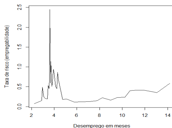
Gráfico 4: Função de Risco (valores medianos das covariáveis).
