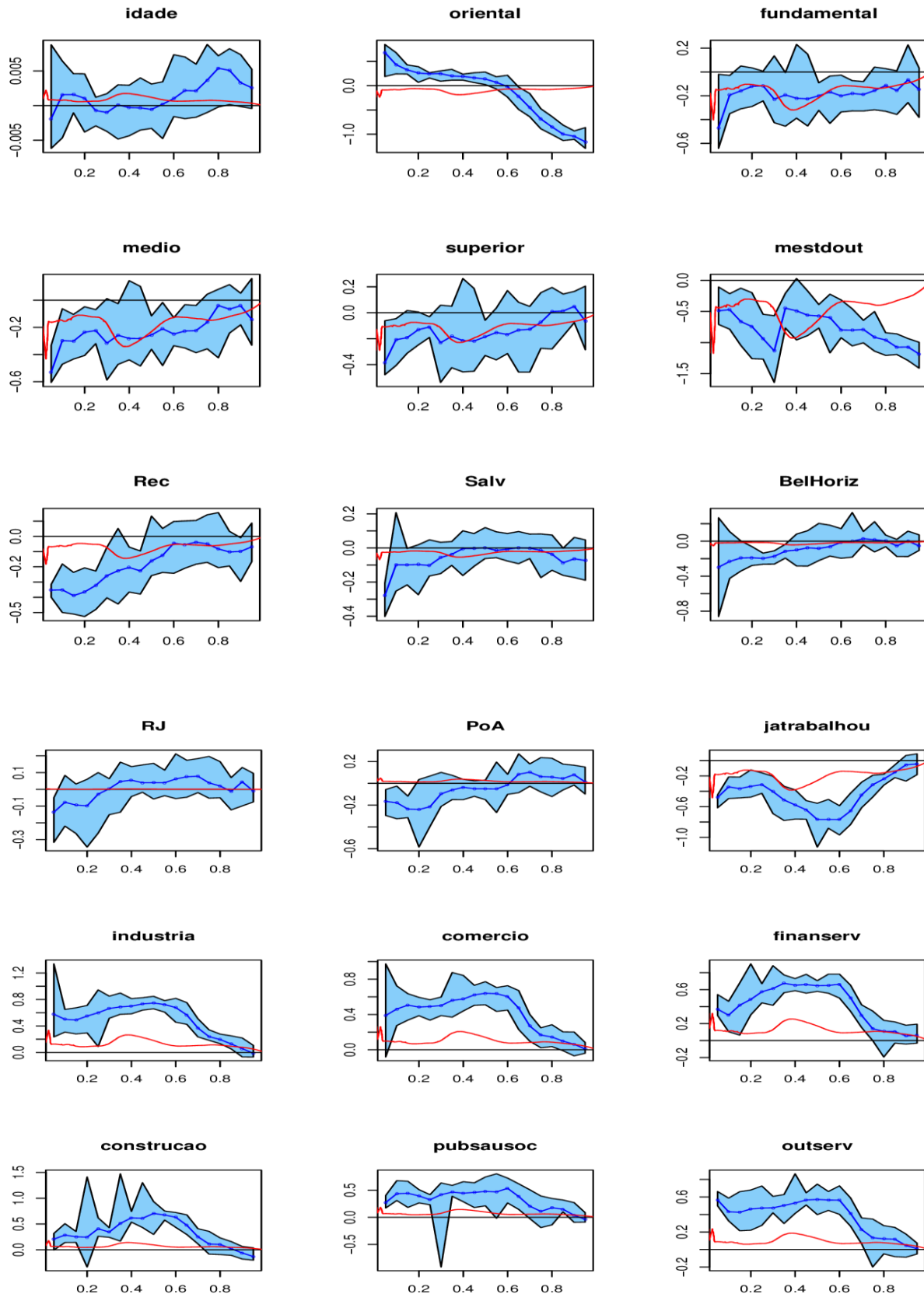
Gráfico 1: Quantis de regressão \beta(\tau) no modelo de regressão quantílica censurada (e intervalo de 95% de confiança por bootstrap ) em azul e o efeito quantílico de tratamento no modelo de Cox (em vermelho).
