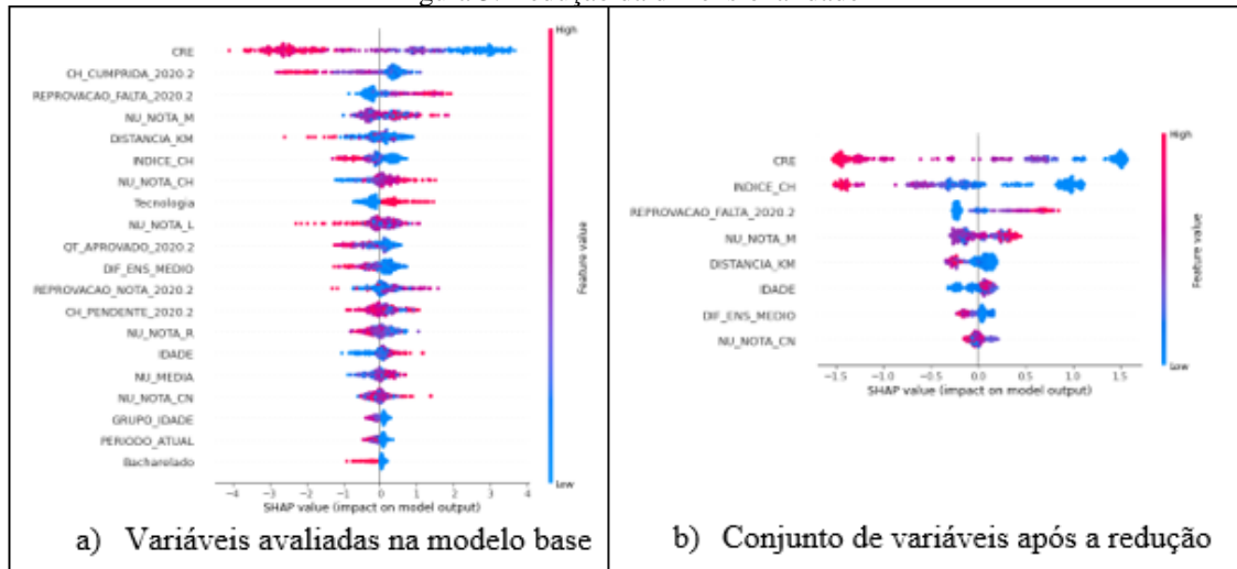
Figura 3: Redução da dimensionalidade
