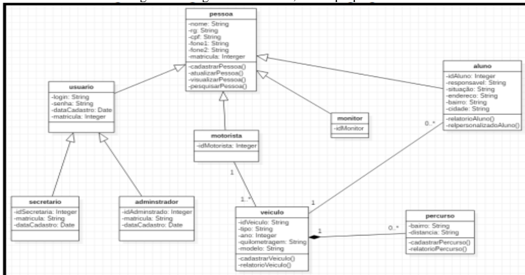
Figura 7 - diagrama de classes, fonte: próprio autor
