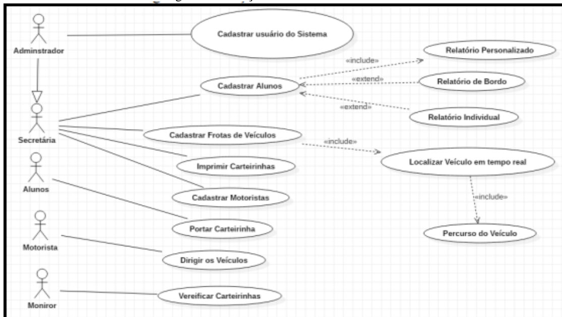
Figura 6 – Relação entre os atores do sistema
