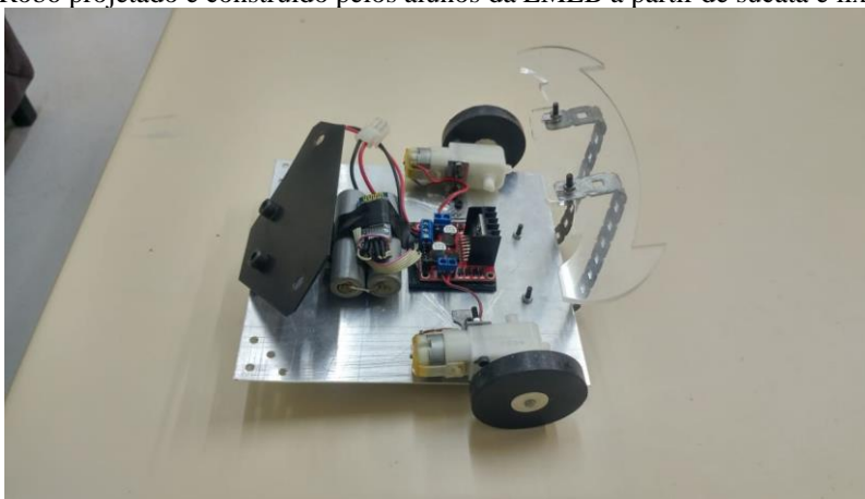
Figura 4 – Robô projetado e construído pelos alunos da EMEB a partir de sucata e lixo eletrônico.
