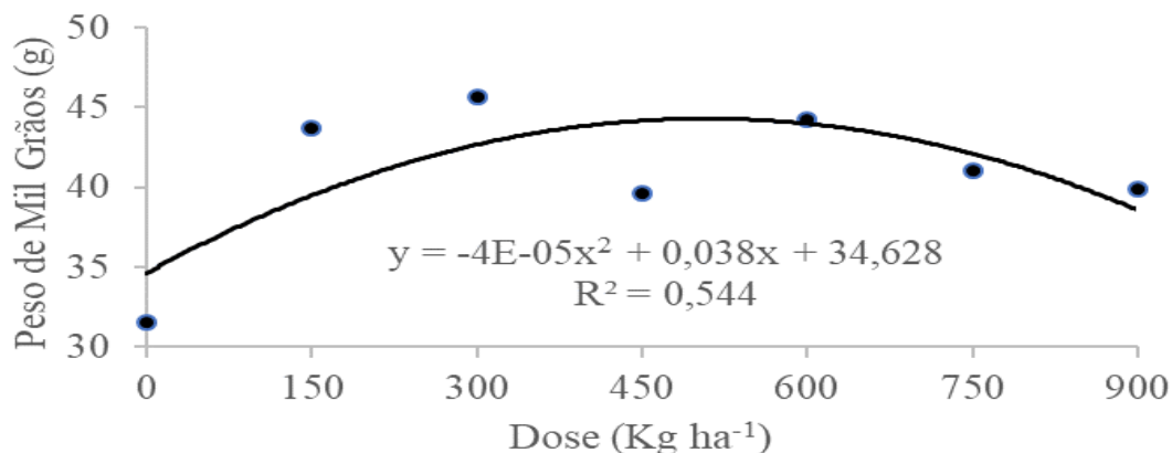
Figura 4 Curva polinomial para variável tecnológica peso de mil grãos na cultura de sorgo, cultivar BUSTER, em função das doses crescente do fertilizante organomineral 04-14-08, nas dose T1: zero Kg ha -1 , T2: 150 Kg ha -1 , T3: 300 Kg ha -1 , T4: 450 Kg ha -1 , T5: 600 Kg ha -1 , T6: 750 Kg ha -1 e T7: 900 Kg ha -1 . Área experimental do Núcleo de Estudo e Pesquisa em Fitotecnia, Mineiros estado de Goiás, 2017.
