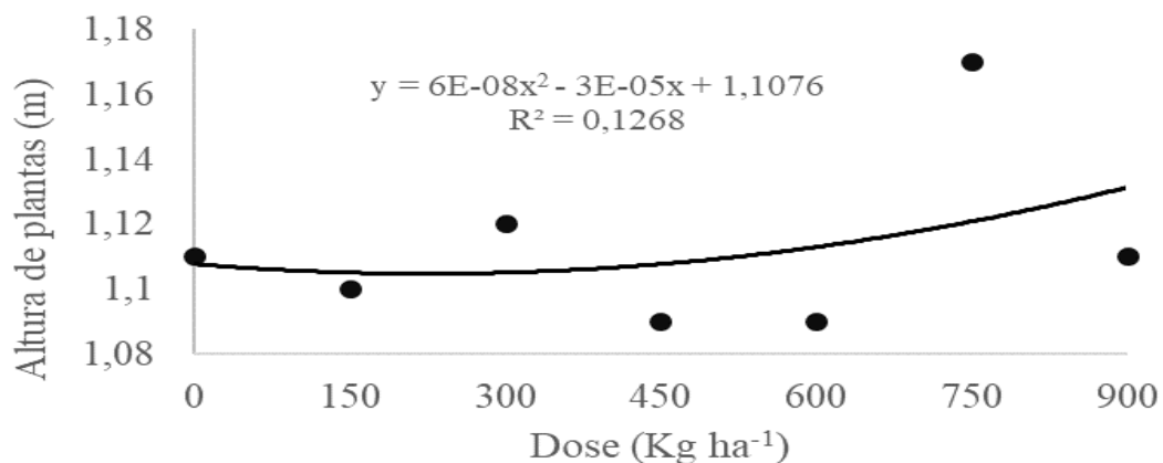
Figura 1. Curva polinomial para variável tecnológica altura de plantas por metro na cultura de sorgo, cultivar BUSTER, em função das doses crescente do fertilizante organomineral 04-14-08, nas dose T1: zero Kg ha -1 , T2: 150 Kg ha -1 , T3: 300 Kg ha -1 , T4: 450 Kg ha -1 , T5: 600 Kg ha -1 , T6: 750 Kg ha -1 e T7: 900 Kg ha -1 . Área experimental do Núcleo de Estudo e Pesquisa em Fitotecnia, Mineiros estado de Goiás, 2017,
