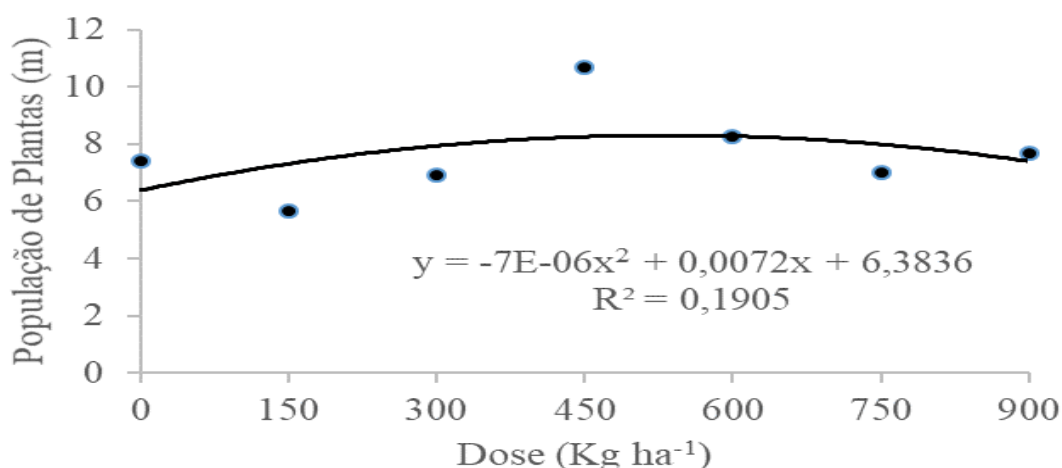
Figura 2. Curva polinomial para variável tecnológica para população de plantas por metro na cultura de sorgo, cultivar BUSTER, em função das doses crescente do fertilizante organomineral 04-14-08, nas dose T1: zero Kg ha -1 , T2: 150 Kg ha -1 , T3: 300 Kg ha -1 , T4: 450 Kg ha -1 , T5: 600 Kg ha -1 , T6: 750 Kg ha -1 e T7: 900 Kg ha -1 . Área experimental do Núcleo de Estudo e Pesquisa em Fitotecnia, Mineiros estado de Goiás, 2017.
