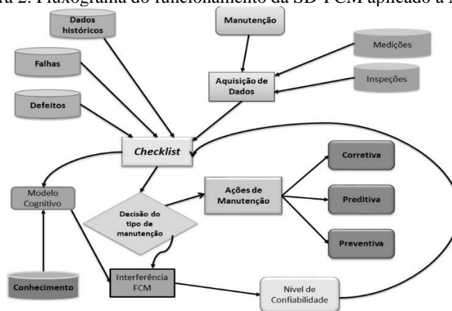
Figura 2. Fluxograma do funcionamento da SD-FCM aplicado a MCC.
