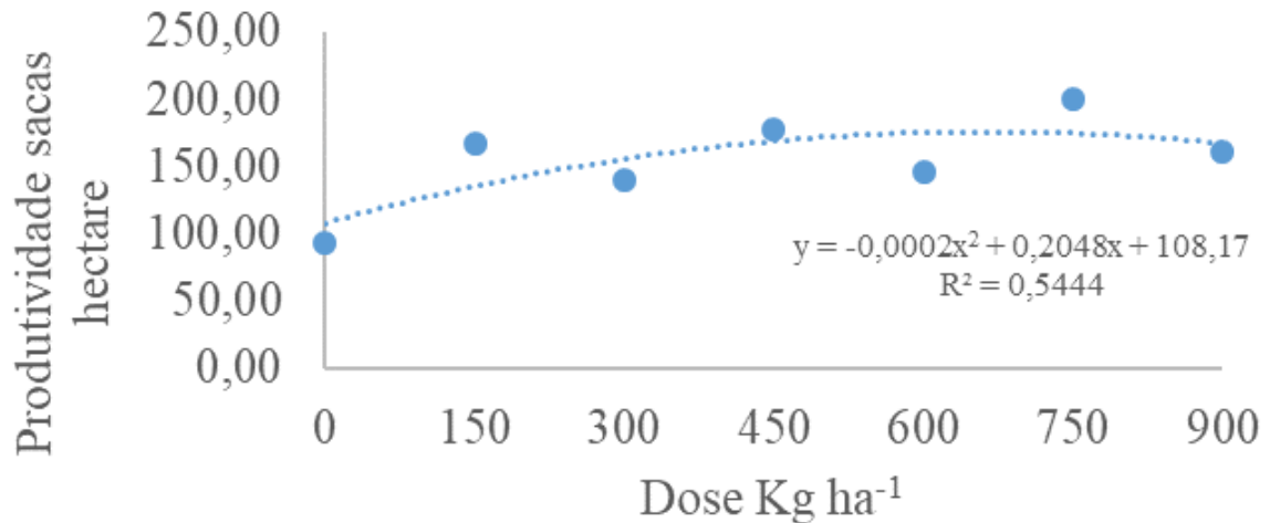
Figura 3 Curva polinomial para variável tecnológica produtividade em sacas por hectare na cultura de sorgo, cultivar MSM 221, conduzido na área experimental do Núcleo de Ensino e Pesquisa em Fitotecnia, Mineiros estado de Goiás, 2017. Em função das doses crescentes do fertilizante organomineral 04-14-08, nas doses T1: zero Kg ha -1 , T2: 150 Kg ha -1 , T3: 300 Kg ha -1 , T4: 450 Kg ha -1 , T5: 600 Kg ha -1 , T6: 750 Kg ha -1 e T7: 900 Kg ha -1 .
