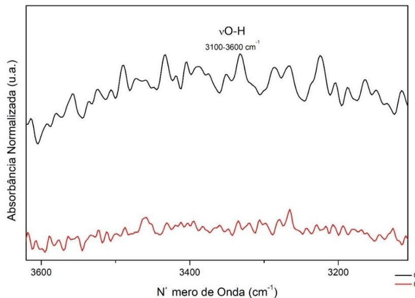
Figura 07 – Espectro ampliado nas bandas entre 3600 \text{cm}^{-1} e 3100 \text{cm}^{-1} do ligante puro CAP 50/70 antes e após o RTFO.
