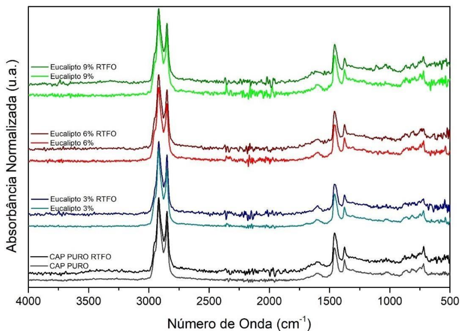
Figura 05 - Espectro dos ligantes puro e modificados com Lignina Eucalipto antes e após o RTFO.
