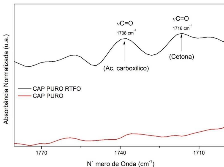
Figura 06 – Espectro ampliado nas bandas 1738 \text{cm}^{-1} e 1716 \text{cm}^{-1} do ligante puro CAP 50/70 antes e após o RTFO.
