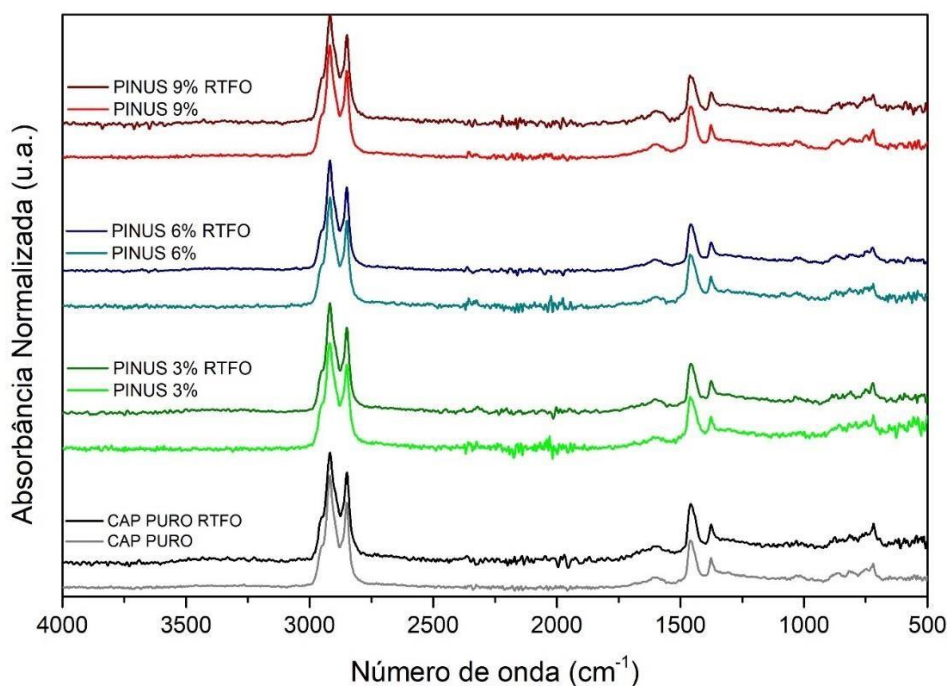
Figura 04 - Espectro dos ligantes puro e modificados com Lignina Pinus antes e após o RTFO.
