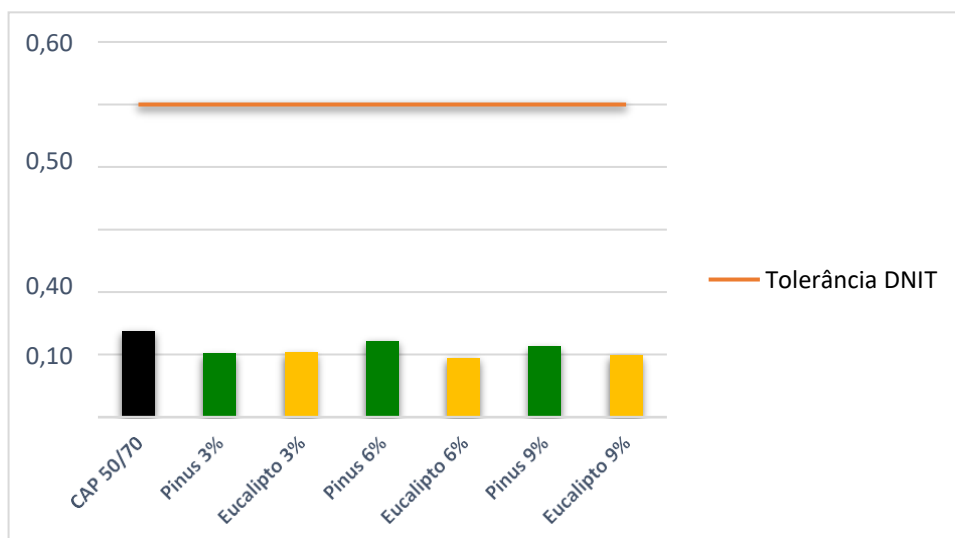
Figura 01 – Perda de massa após RTFO.
