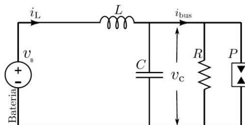
Fig. 3 Configuração da Nanorrede para Q2 está aberto e Q1 conduz.
