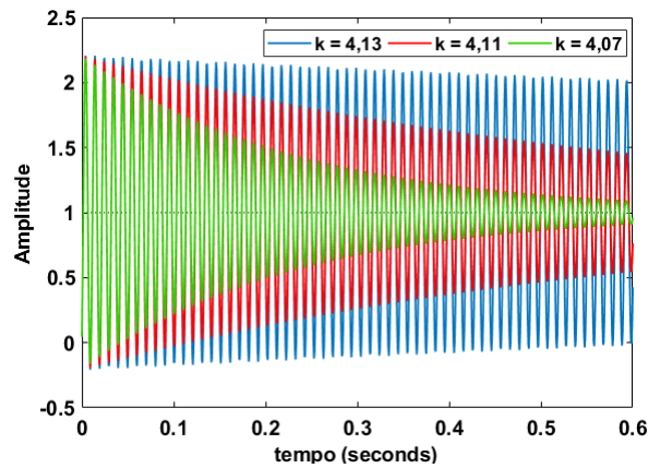
Fig. 6 Resposta ao degrau de T_{MF} para variações de k
