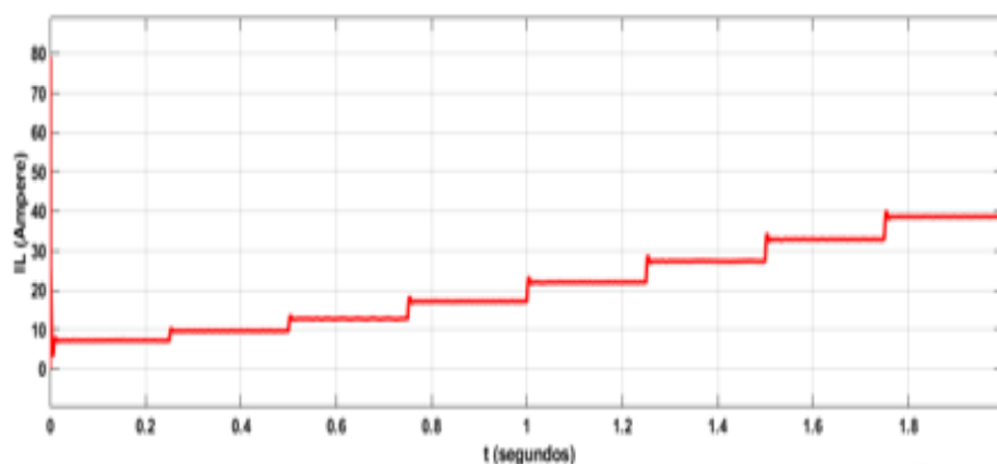
Fig. 8 Resultados para o SIMULINK i_L do barramento
