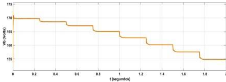
Fig. 9 Resultados para o SIMULINK para a tensão v_B das baterias
