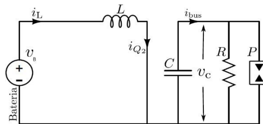
Fig. 2 Configuração da Nanorrede em que Q2 conduz e Q1 está aberto.
