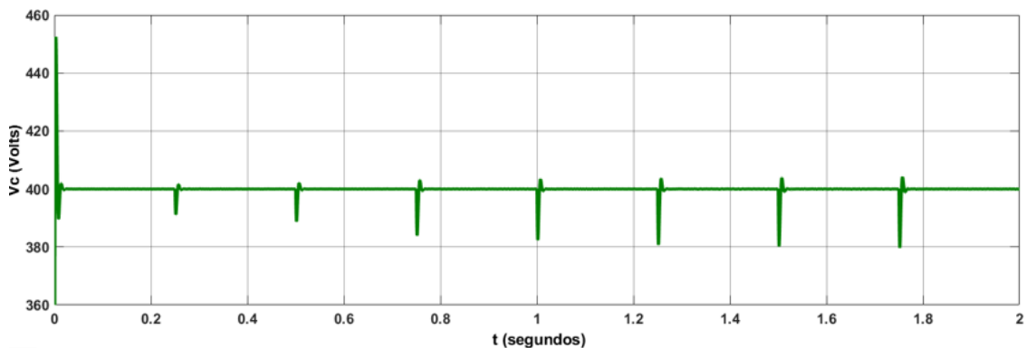
Fig. 10: Resultados para o SIMULINK para tensão v_C do barramento
