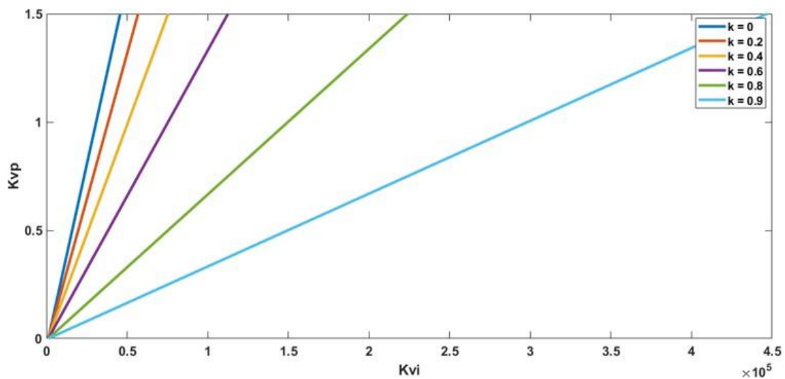
Fig. 5 Variação de k_{vp} em função de k_{vi} para diferentes valores de k
