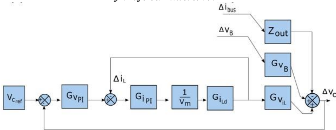
Fig. 4: Diagrama de Blocos do Controle
