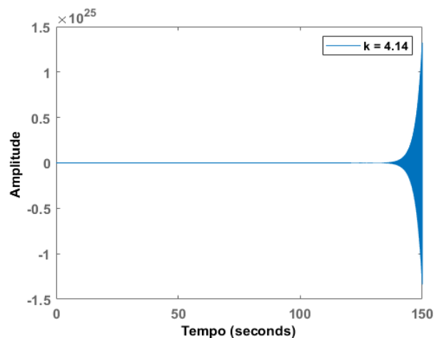
Fig. 7 Resposta ao degrau de T_{MF} para k = 4,14
