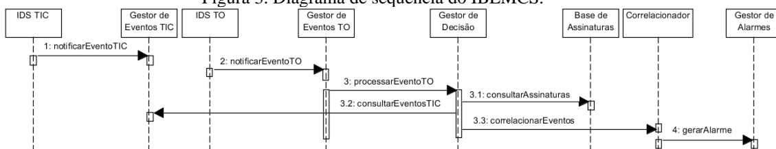
Figura 3. Diagrama de seqüência do IBEMCS.
