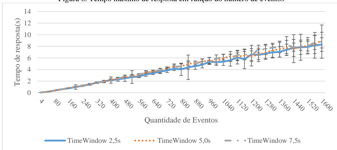
Figura 6. Tempo máximo de resposta em função do número de eventos
