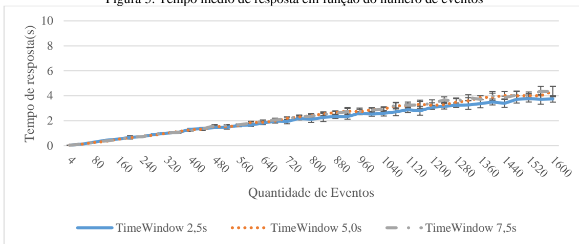
Figura 5. Tempo médio de resposta em função do número de eventos
