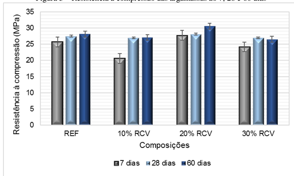
Figura 3 – Resistência à compressão das argamassas ao 7, 28 e 60 dias
