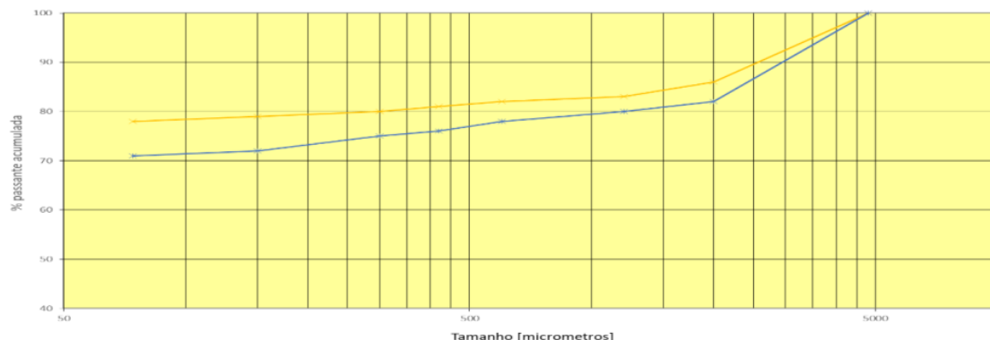
Figura 2. Curva granulométrica de jazidas. Análise Granulométrica
