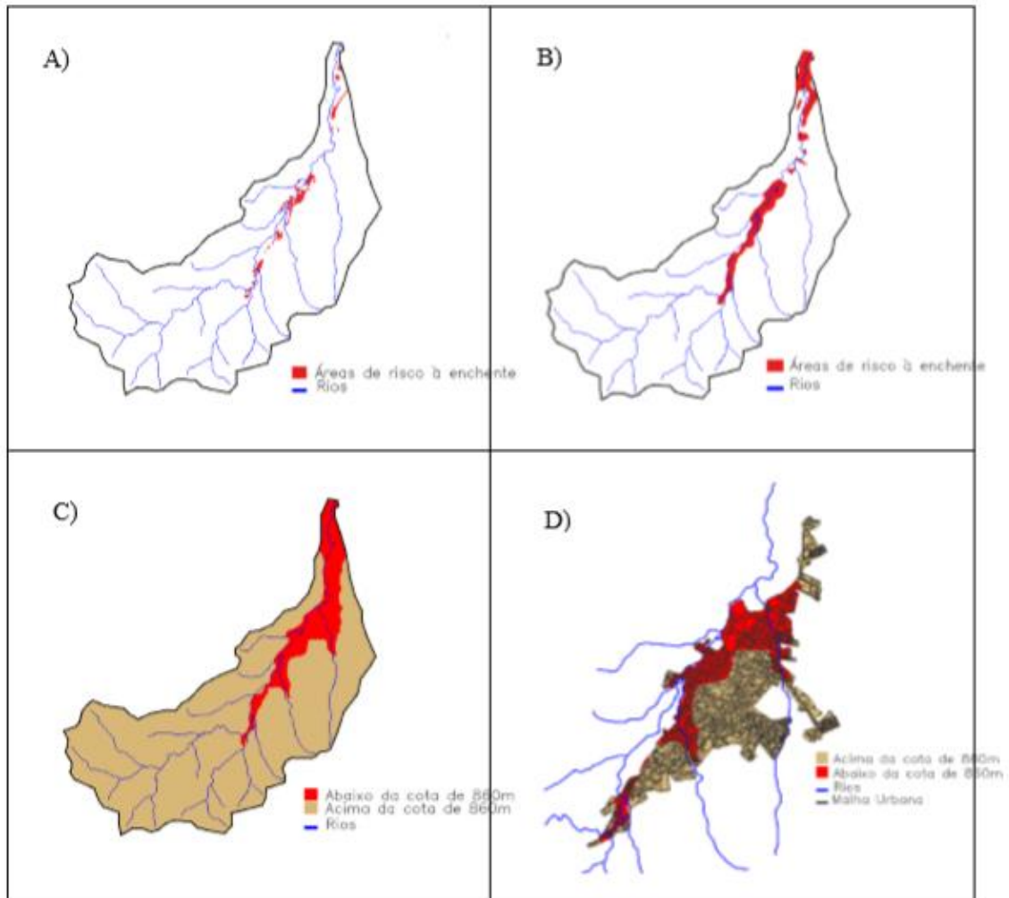
Figura 1. Áreas de Risco à enchentes considerando-se declividade de 0 a 3%, Distância da margem do rio de 0 a 150m, cota de enchente de 860m e níveis de capacidade de infiltração baixo e médio (A); Áreas de Risco à enchentes considerando-se declividade de 0 a 3%, Distância da margem do rio de 0 a 150m e cota de enchente de 860m (B); Áreas abaixo e acima da cota de enchente do ano de 2014 (C); Área urbana da bacia do Rio Faxinal acima e abaixo da cota de enchente do ano de 2014 (D).
