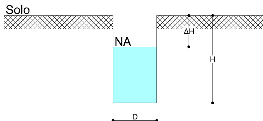
Figura 1 - Ensaio ABGE (1996)
