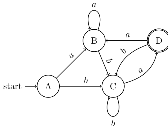
Figura 2.2: DFA dell'esempio 2.1.1
