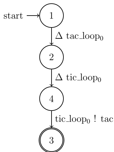
Figura 4.14: Vista locale di start
