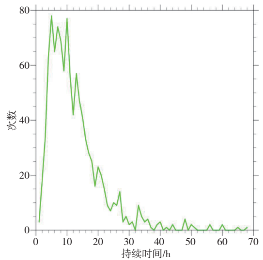
图8 2008—2017年四川省不同持续时间突发性暴雨事件发生的频次
