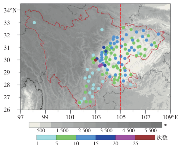
图2 2008—2017年四川省突发性暴雨事件频次的空间分布(彩色圆点表示频次,红色虚线为四川盆地东西部分界线,下同)
