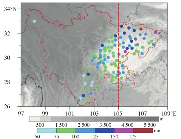
图9 2008—2017年四川省国家站突发性山地暴雨事件的平均累计雨量的空间分布(单位:mm)
