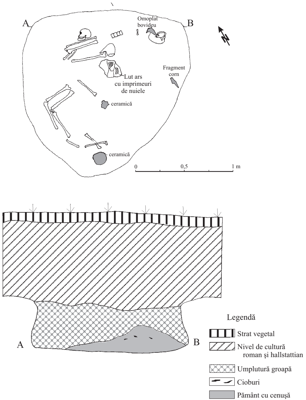
Fig. 1 Groapa 1. Plan și profil. Fig. no 1. La fosse no 1. Plan et profil.
