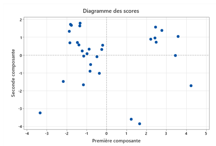
Figure 4 : Diagramme de dispersion des individus
