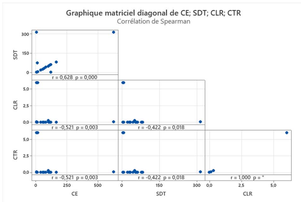
Figure 9 : Matrice diagonale de CE, SDT, CLR, CTR selon la corrélation de Spearman
