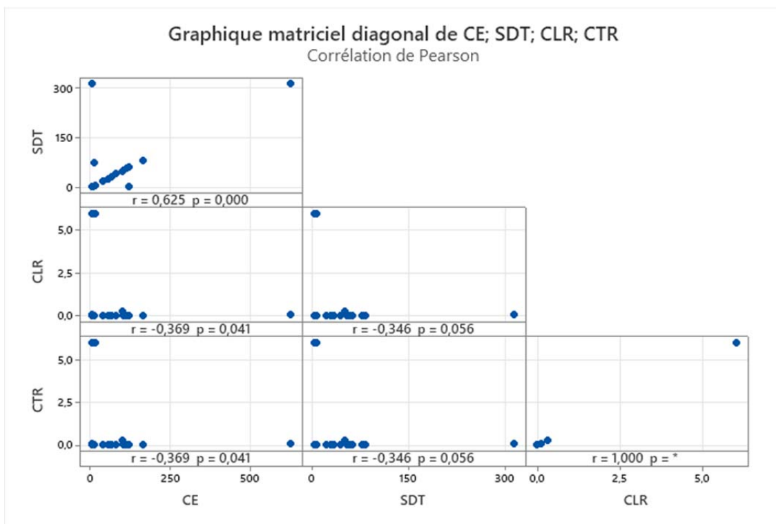
Figure 8 : Matrice diagonale de CE, SDT, CLR, CTR selon la corrélation de Pearson
