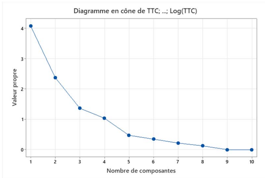
Figure 3 : Nombre de composantes principales par rapport à leurs valeurs propres
