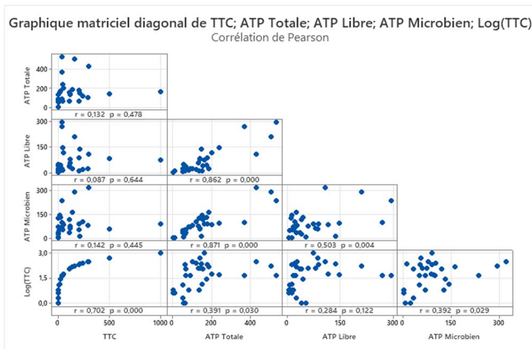
Figure 6 : Matrice diagonale de TTC, ATP Total, ATP Libre, ATP Microbien, Log (TTC) selon la corrélation de Pearson
