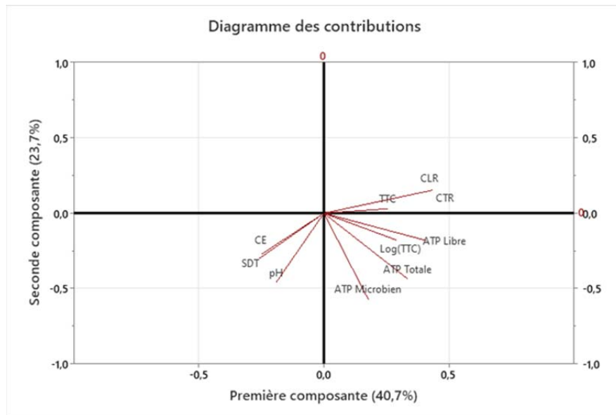
Figure 5 : Diagramme des contributions des variables
