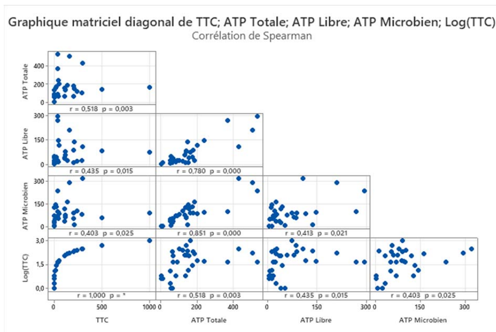
Figure 7 : Matrice diagonale de TTC, ATP Total, ATP Libre, ATP Microbien, Log (TTC) selon la corrélation de Spearman
