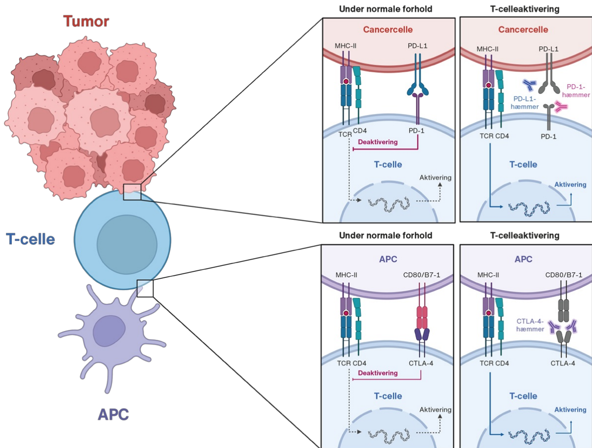
FIGUR 1 Skitsering af, hvordan T-celler kan aktiveres til at eliminere cancerceller. Under normale forhold vil bindingen mellem programmeret death-ligand 1 (PD-L1) på en cancer-celle og programmeret death-protein 1 (PD-1) på en T-celle føre til et genkendelses- og overlevelsessignal mellem T-cellen og cancercellen. Når dette signal blokeres vha. PD-L1-hæmmere (f.eks. atezolizumab, avelumab) eller PD-1-hæmmere (f.eks. pembrolizumab, nivolumab, dostarlimab) aktiveres T-cellen til at destruere cancercellen. Endvidere vil bindingen mellem cluster of differentiation 80 (B7-1) på antigenpræsenterende celler og cytotoxisk T-celleassocieret antigen 4 (CTLA-4) på T-celler under normale forhold holde immunforsvaret i skak. Blokering af dette signal vha. CTLA-4-hæmmere (f.eks. ipilimumab, tremelimumab) fører til aktivering og rekruttering af T-celler, som kan destruere cancerceller. Figuren er udarbejdet på BioRender.com.
