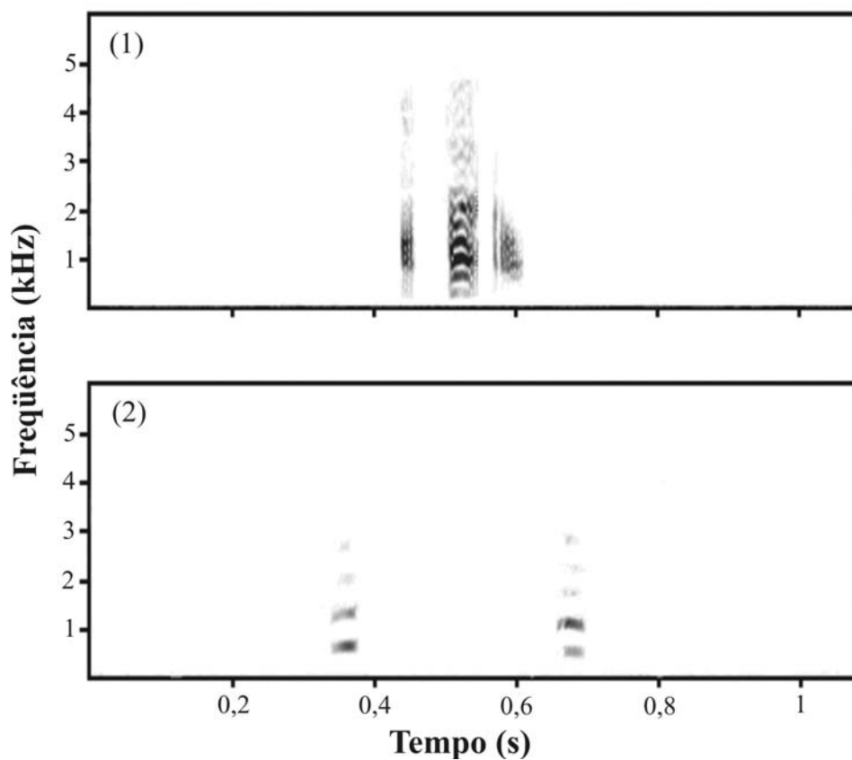
Hyla semilineata Spix, 1824 (MNRJ 29764, temperatura do ar 23,2°C): fig.1- sonograma do canto de anúncio, fig.2- sonograma do canto de encontro.
