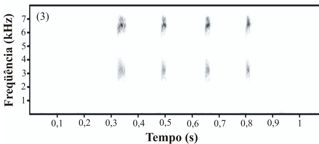
Fig.3- Sonograma do canto de anúncio de Hyla wernerii (MNRJ 30401, temperatura do ar 23,7°C)
