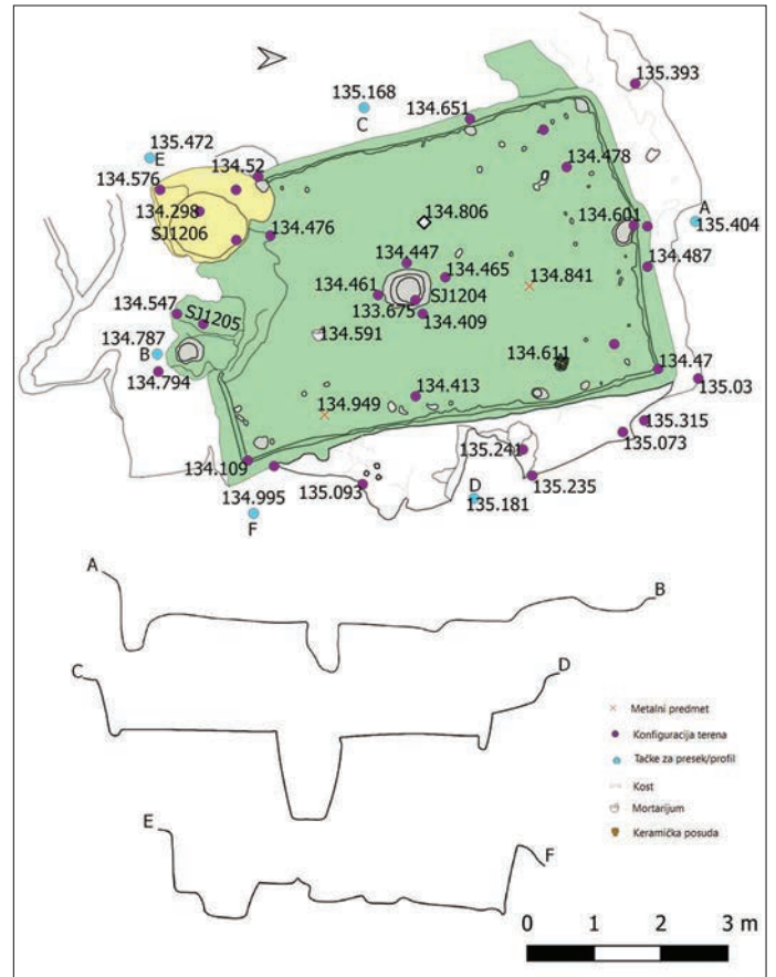
Слика 8. Основа и пресеци куће 4, нацртала И. Кајтез, документација Међуопштинског завода за заштиту споменика културе Суботица Figure 8. Ground plan and cross-sections of house 4, drawn by I. Kajtez, Documentation of the Intermunicipal Institute for the Protection of Cultural Monuments Subotica
