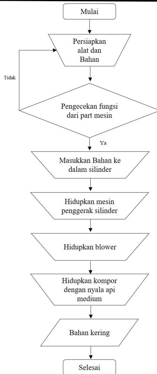
Gambar 5. Tahapan Pengoperasian Mesin Pengering Kopi
