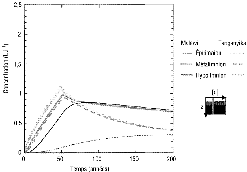
Figure 5 Évolution temporelle des concentrations dissoutes en un élément de type CI dans les différents compartiments des lacs Malawi et Tanganyika en réponse à une pollution chronique véhiculée sous forme dissoute par les affluents pendant 50 ans.
