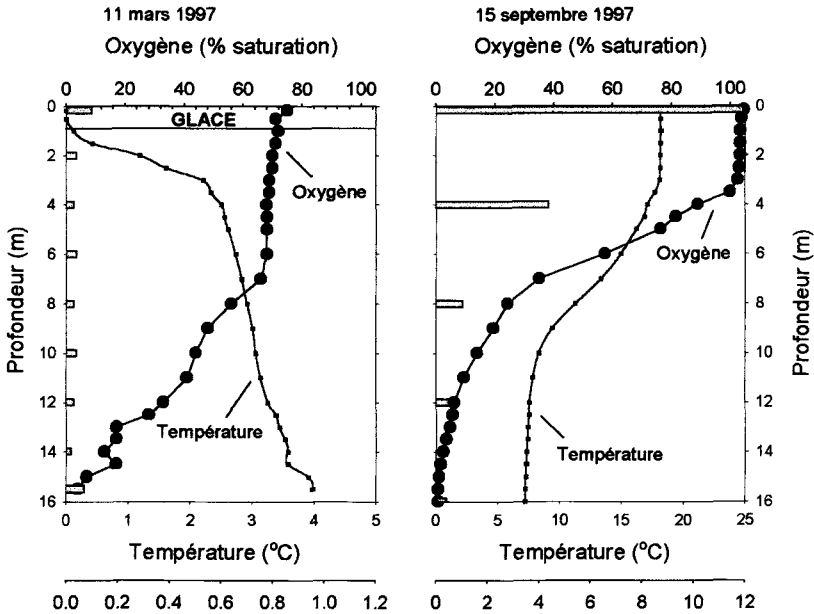
Figure 3 Diminution des concentrations en oxygène dans les couches inférieures de la colonne d'eau du lac Saint-Charles à la fin de la stratification hivernale (a, 11 mars 1997) et estivale (b, 15 septembre 1997). Les profils de température (petits carrés) et d'oxygène (grands cercles), de même que les valeurs de chlorophylle a (barres) proviennent de la région la plus profonde du bassin nord. À noter la différence des échelles de température et de chlorophylle a entre les deux graphiques.
