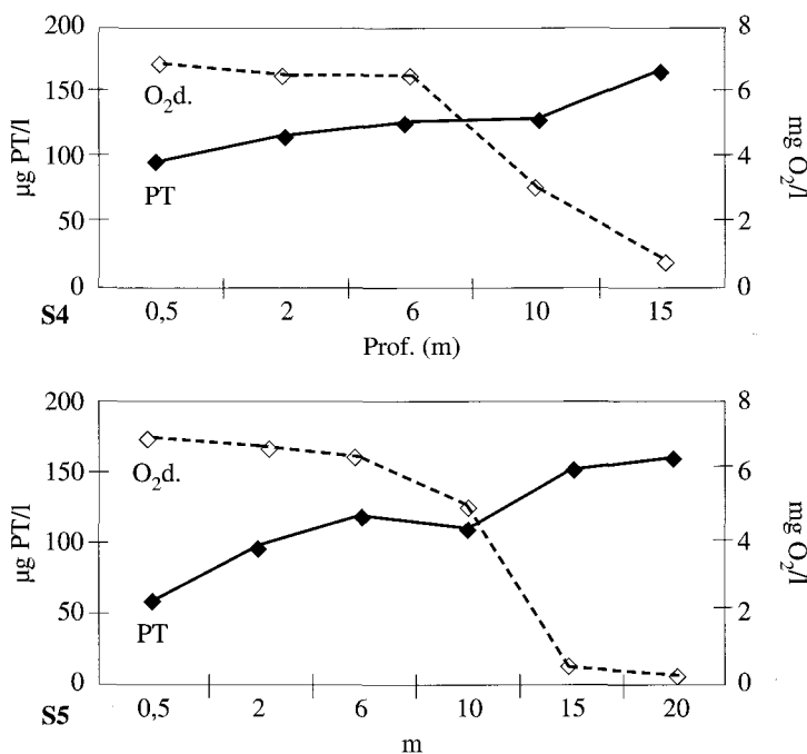
Figure 2 Évolution verticale du phosphore total (PT) et de l'oxygène dissous ( \text{O}_2\text{d} ) aux stations S4 et S5 durant la campagne estivale.
