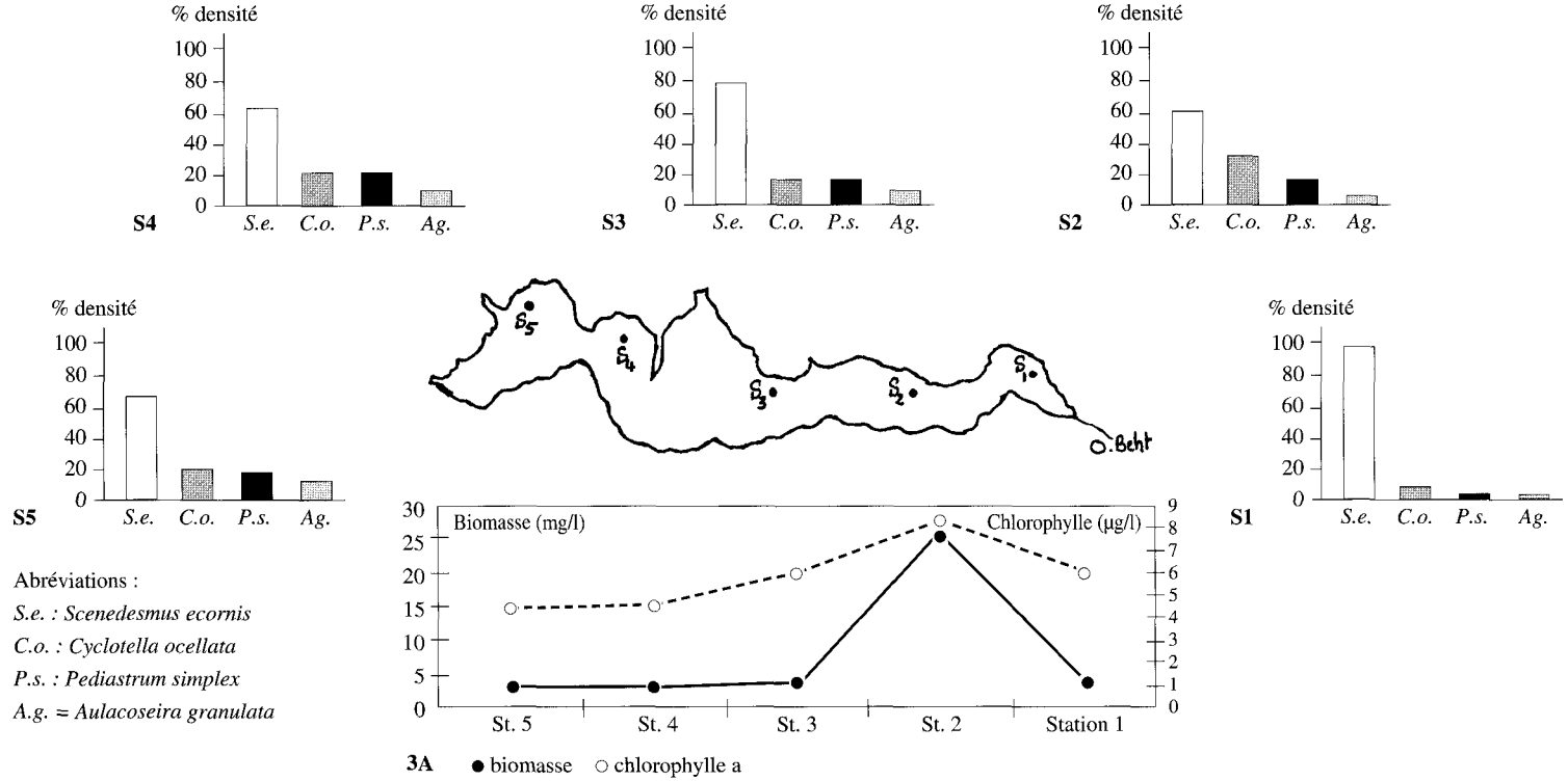
Figure 3 Distribution longitudinale de la biomasse algale (poids frais) et de la chlorophylle a (3A) et des % de densité des principales espèces dans les différentes stations de la retenue, durant la campagne printanière (valeurs moyennes de la colonne d'eau). Longitudinal distribution of alga biomass (wet weight) and chlorophyll a (3A) and % of density of principal species at different stations of the lake, during the spring campaign (mean values on total water column).
