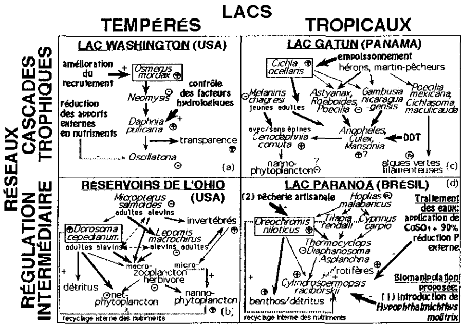
Figure 4 Cas types de réseaux trophiques à cascades trophiques ou régulation intermédiaire dans les lacs tempérés et tropicaux. Les effets de la prédation et du broutage sont indiqués par des flèches dont la grosseur est proportionnelle à l'intensité des effets. Les stimulations sont indiquées par des signes « + » et les réductions par des signes « - ». Les altérations naturelles et les manipulations anthropiques sont indiquées en lettres grasses et par des flèches épaisses. Les apports externes et les recyclages internes en nutriments sont matérialisés par des flèches en grisé. Les espèces piscicoles clés au sommet de la chaîne trophique (cascades) ou au centre du réseau trophique (régulation intermédiaire) sont encadrées. Cas types : a : Lac Washington, États-Unis, lac tempéré, cascades trophiques ; b : réservoirs plats de l'Ohio, États-Unis, milieux tempérés, régulation intermédiaire ; c : Lac Gatun, Panama, lac tropical, cascades trophiques ; d : Lac Paranoá, Brésil, lac tropical, régulation intermédiaire. Voir détails et références dans le texte.
