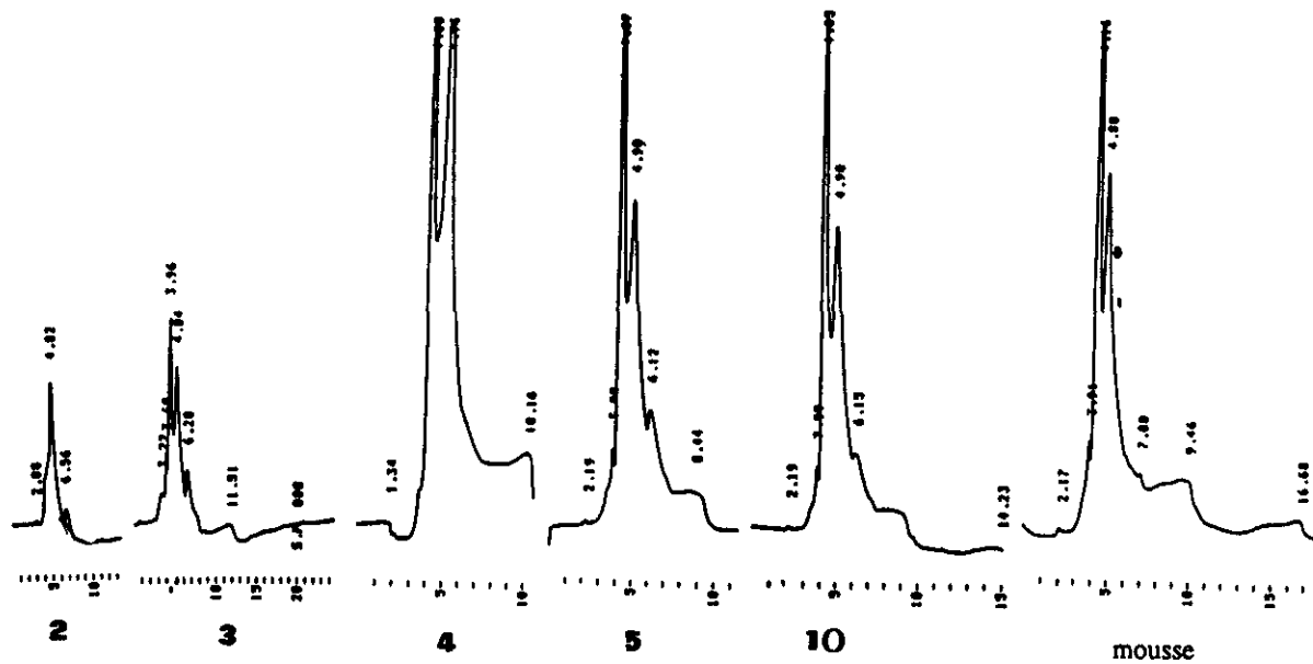
Figure 6 Chromatogrammes HPLC de l'Eau de la Vienne en fonction des points de prélèvement. Campagne du 1 er octobre 1991. HPLC chromatography of Vienne water versus sampling points. Sampling campaign of Oct. 1, 1991.
