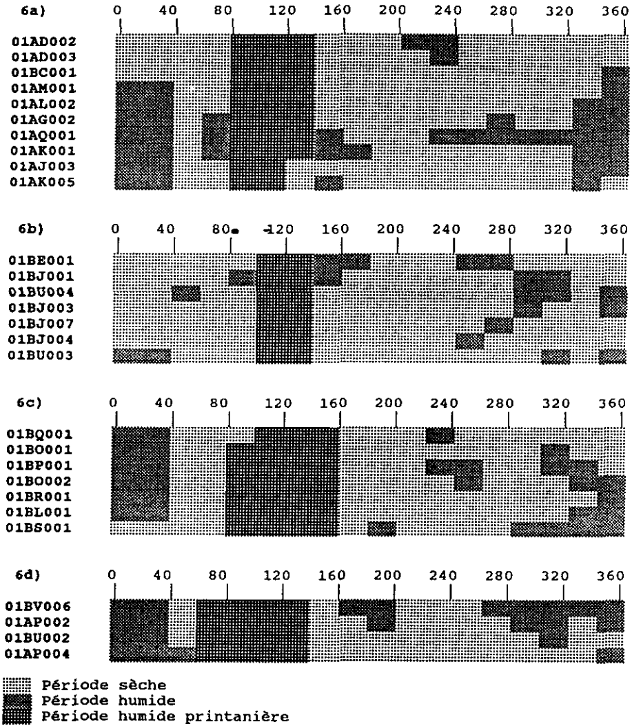
Figure 6 Illustration des régions homogènes du N.B.
