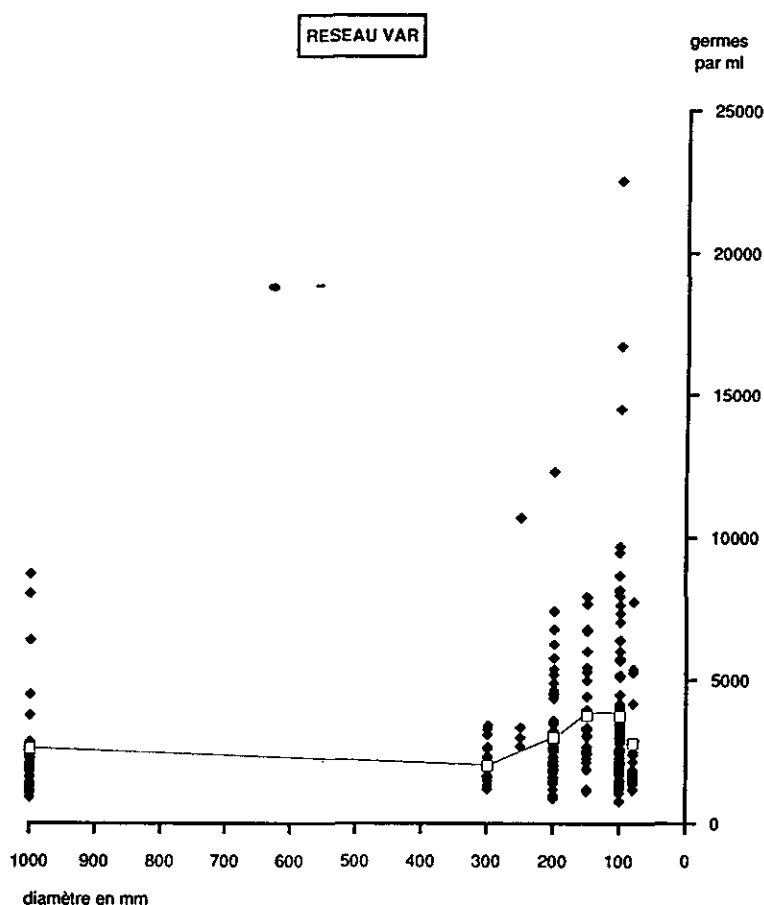
Figure 5 Réseau Var : germes totaux par épifluorescence en fonction du diamètre des canalisations.
