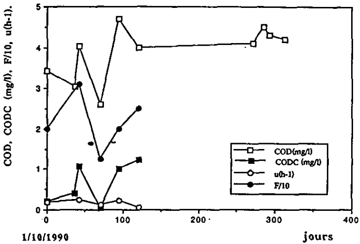
Figure 2 Evolution de la qualité de l'eau brute en fonction du temps : COD, CODC, F, U.
