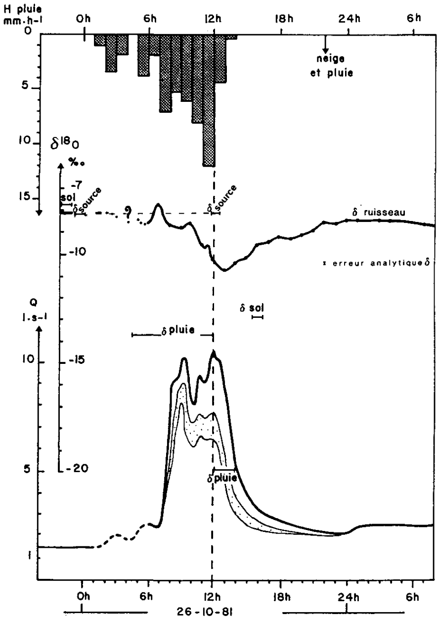
Figure 2 La crue du 26-10-81. Limnigramme et hyétogramme. Composition isotopique des eaux de pluie, du sol, de la source et de la rivière avant et pendant la crue.
