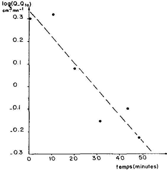
Figure 5.- Etude de la vidange du réservoir en relation avec le suintement L3 (débit total Q diminué au débit stabilisé Q_{\infty} = 4 \text{ cm}^3.\text{mn}^{-1} ) à la suite de la cassure des produits de colmatage (l'origine des temps est prise à l'instant de la cassure). Cette vidange s'ajuste selon une loi :
