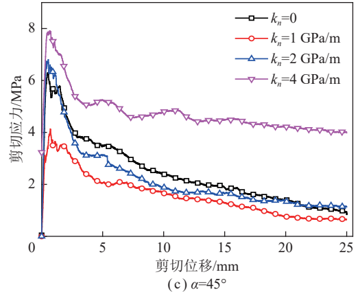
图 4 剪切应力-剪切位移曲线
