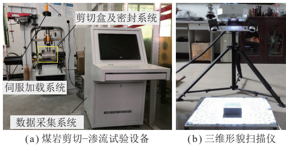
图 3 试验系统
