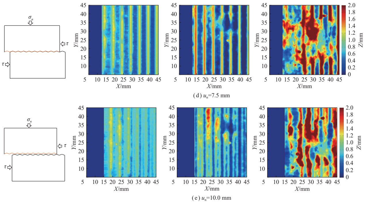
图 13 结构面动态破坏过程
