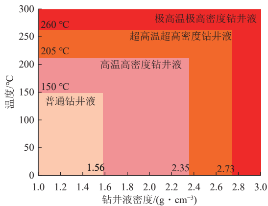
图 2 钻井液体系适应的温度与密度范围的界定 [17]
