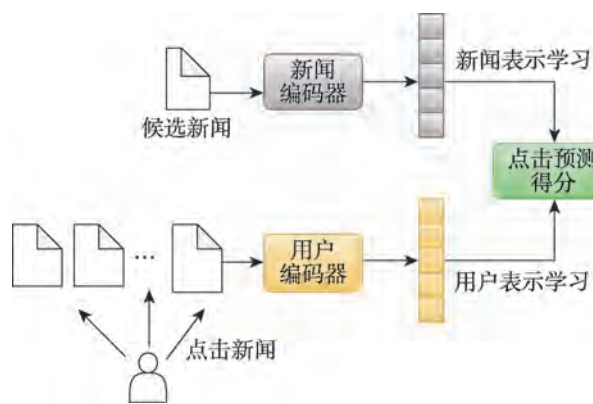
图2 新闻-用户表示学习框架
