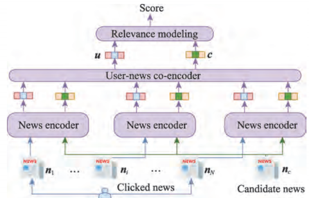
图 9 KIM 模型的结构
