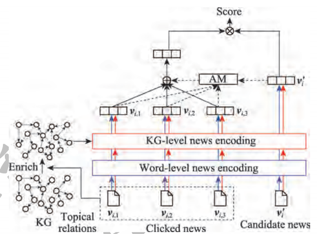
图7 TEKGR模型的结构
