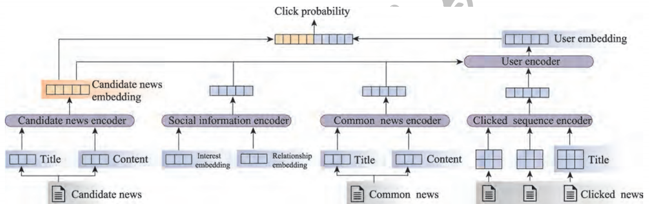
图 10 SI-News 模型的结构
