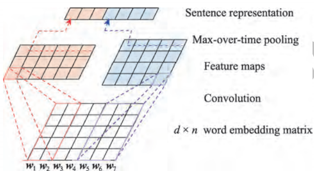
图6 KCNN结构
