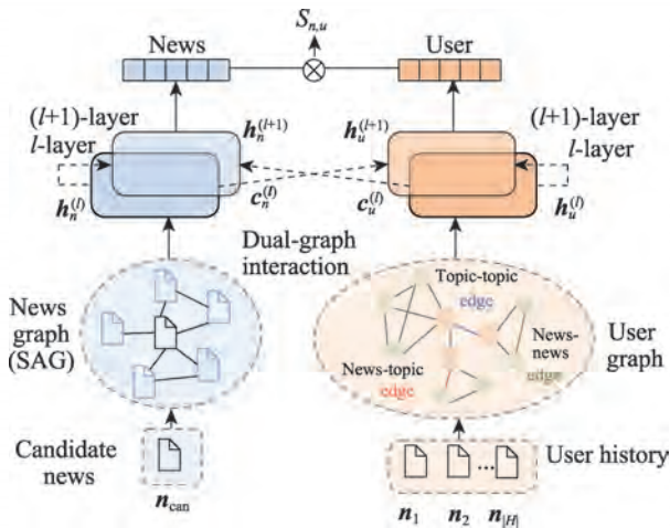
图5 DIGAT结构
