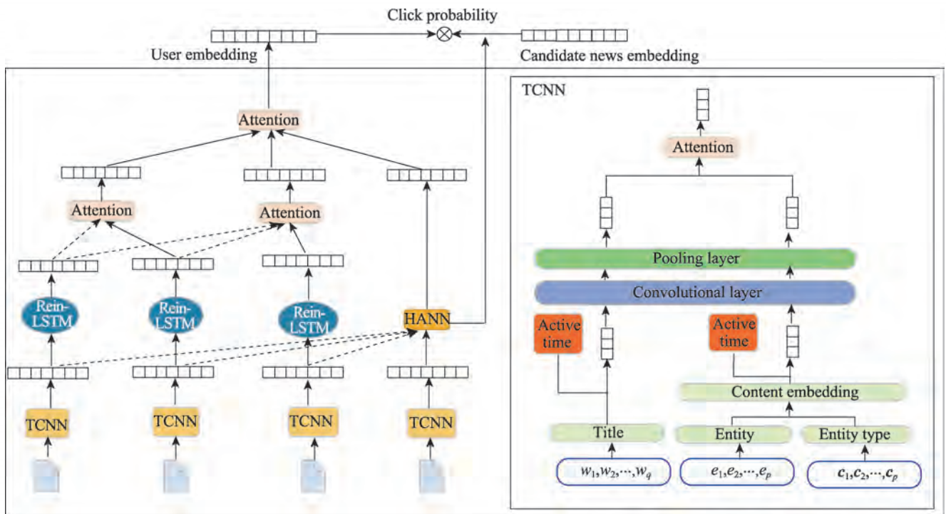
图4 TSHGNN 结构
