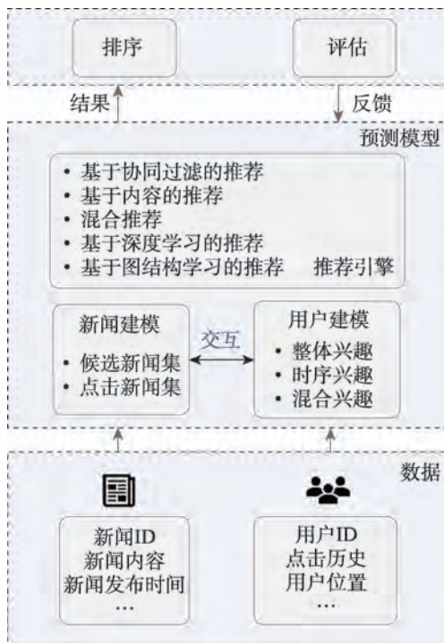
图1 个性化新闻推荐系统架构
