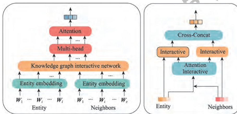
图 8 NRKM 实体编码器和 KGIN 结构
