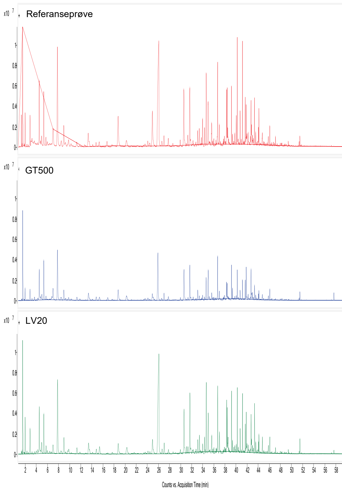
Figur 4 Gasskromatogram av melprøve uten antioksidant (Referanseprøve), med 500 ppm Guardian Toco 70 (GT500), og 20 % limvann (LV20). 1: Trimetylammin, 2: 2-metyl-furan, 3: 2-butanon, 4: 2-etyl-furan, 5: 2-metyl-2-butenal, 6: 2-metyl-2-pentenal, 7: 1-penten-3-ol, 8: 2-pentyl-furan, 9: 3-etyl-4-metyl-heksan, 10: 2-cis, 2-penten-1-ol, 11: 2-nonanon, 12: 1-okten-3-ol, 13: ukjent aromat, 14: tr,cis,3,5-Oktadien-2-on.
