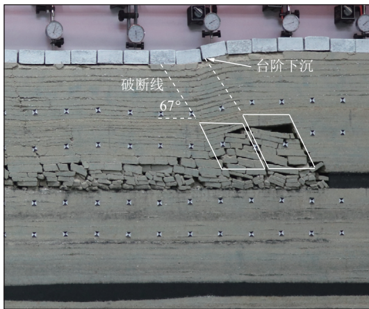
图3 上煤层开采承载岩层“台阶岩梁”结构
