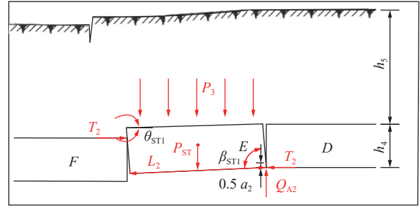
图 12 上煤层“台阶岩梁”结构力学计算模型
