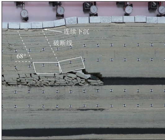
图2 上煤层开采承载岩层“铰接岩梁”结构
