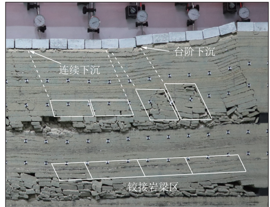
图4 下煤层开采承载岩层结构
