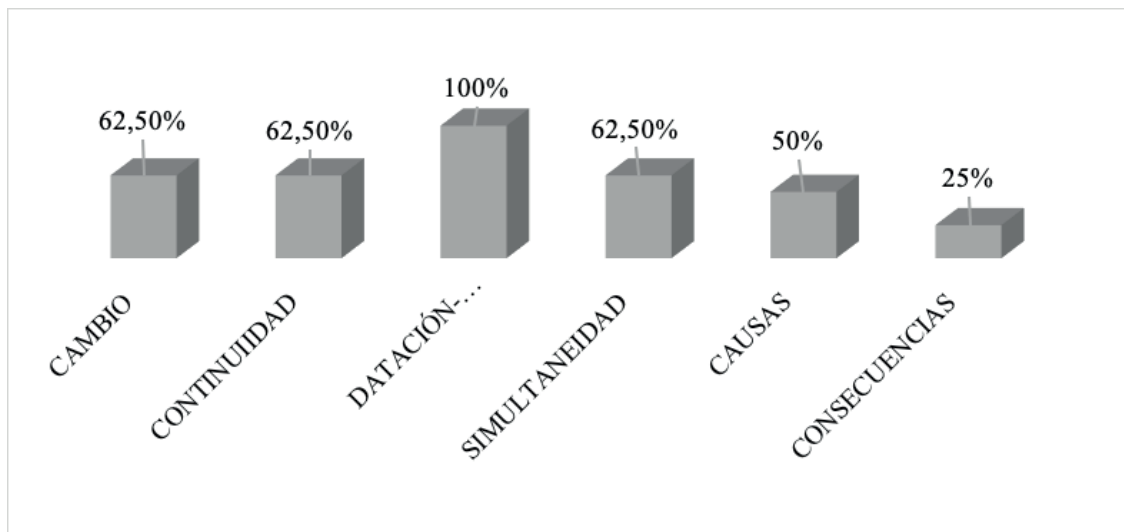
Figura 3. Operadores temporales
