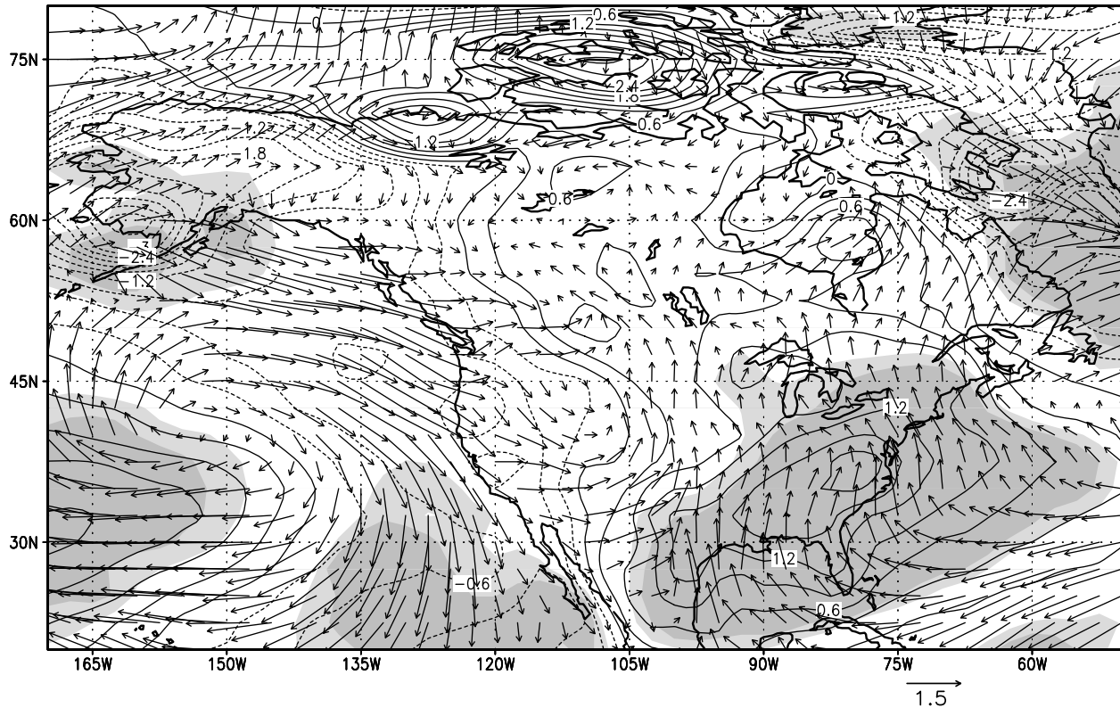
(d) -NAO/La Nina (state 4)
