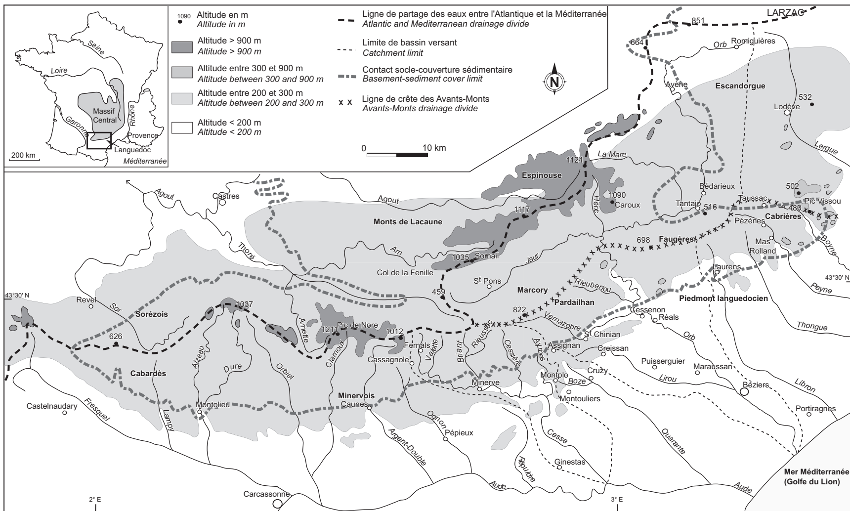
FIGURE 1. Carte de localisation et topographie régionale de la Montagne Noire. Location map and topography of the Black Mountain region.
