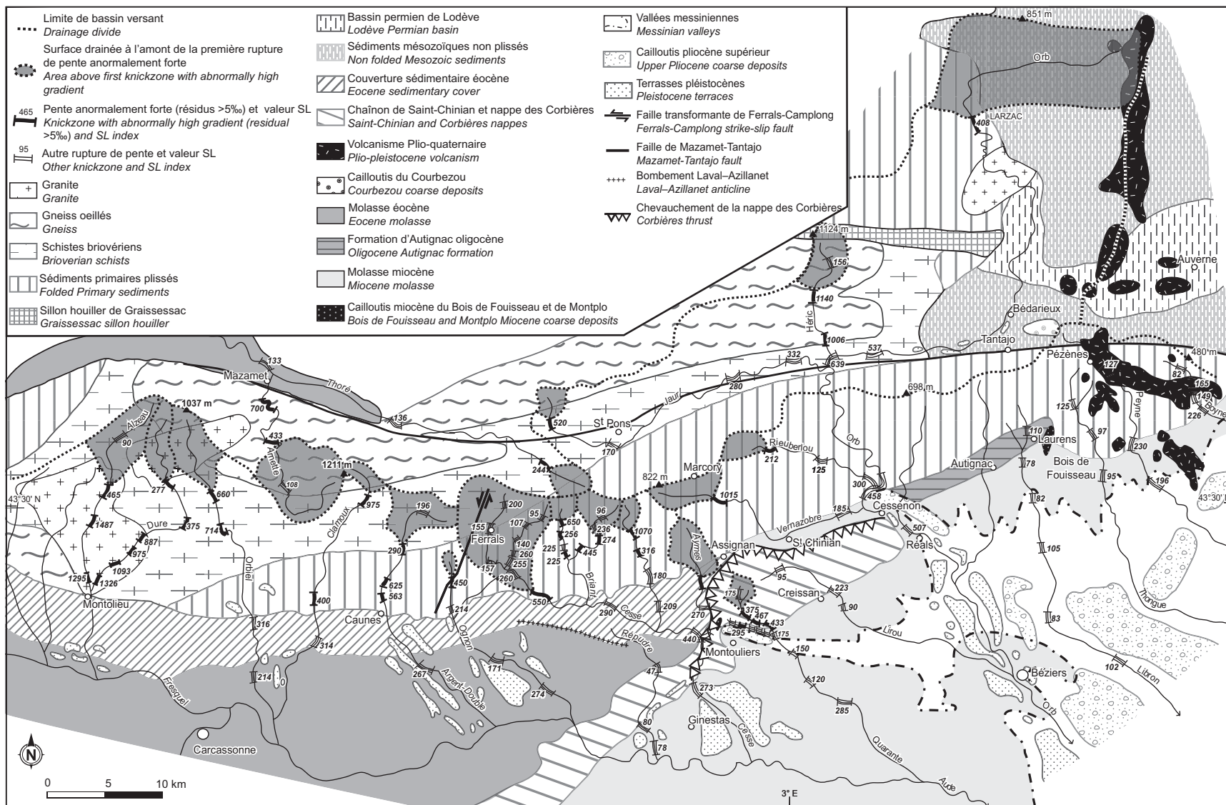
FIGURE 2. Cadre morphostructural, ruptures de pente et dépôts corrélatifs de l'érosion. Morphostructural map, knickzones and detrital deposits.
