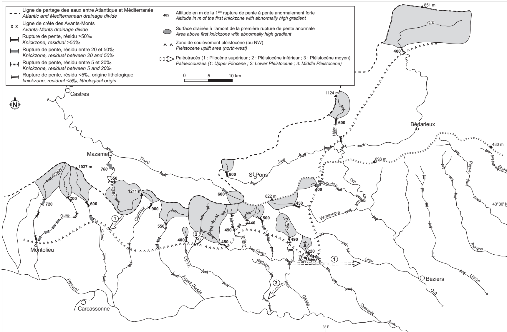
FIGURE 9. Localisation des ruptures de pente à pente anormalement forte (résidus >5 ‰) et des zones de soulèvement pléistocène. Location of knickzones with abnormally high gradient (residual >5 ‰) and of Pleistocene uplift areas.
