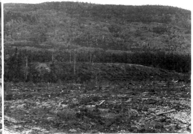
FIGURE 19. Front d'une accumulation en nappe de débâcle glaciaire. Il est perpendiculaire au sens de l'écoulement et légèrement sinueux. Front of an outburst deposit. It is perpendicular to flow direction and slightly sinuous.
