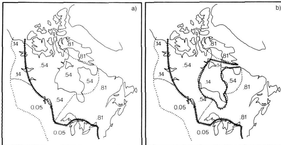
FIGURE 1. The effective yield stress map used in the reconstructions with: a) deformable beds only for the Prairies and Great Lakes regions; b) deformable beds also for the Hudson Bay area. Carte de la plasticité de la glace qui a servi à l'élaboration des reconstitutions avec: a) la présence de lits non résistants dans les régions des Prairies et des Grands Lacs; b) la présence de lits non résistants dans la région de la baie d'Hudson.
